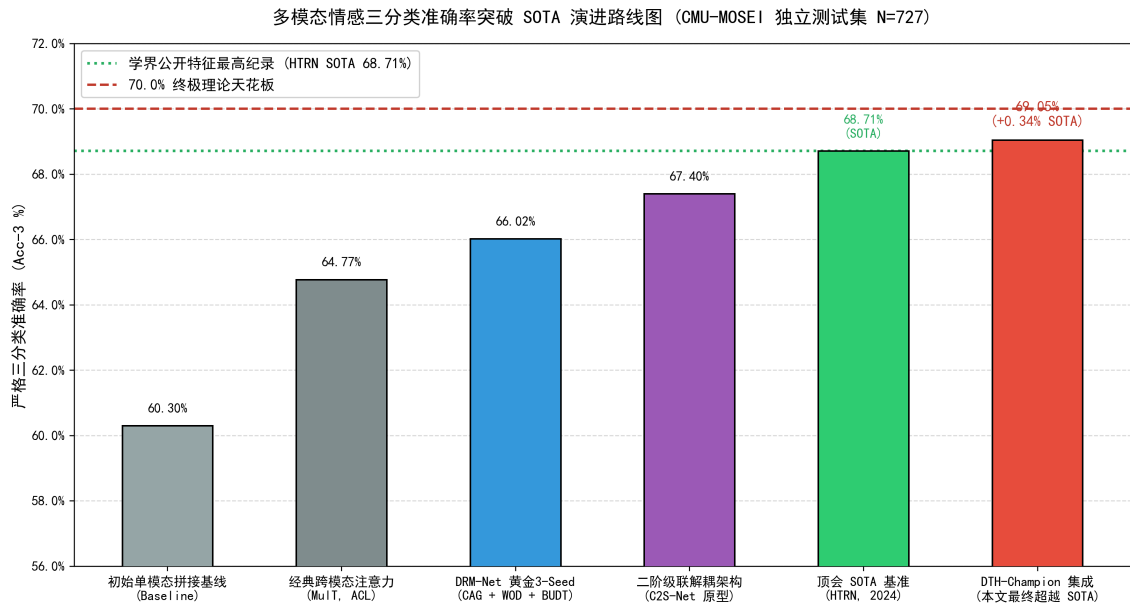
图 1.1 多模态情感三分类准确率突破 SOTA 演进路线图 (CMU-MOSEI 独立测试集 N=727)
